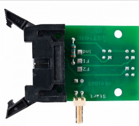
Snímač hriadeľa - CNY-70 s prídavným konektorom
